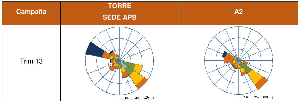
Figura 3. Rosas de viento durante las campañas.
