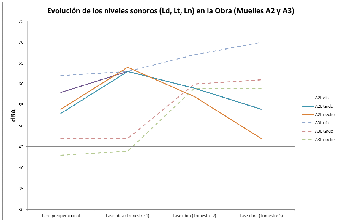
Figura 4. Evolución de los niveles de ruido en el desarrollo de la obra (Muelles)
