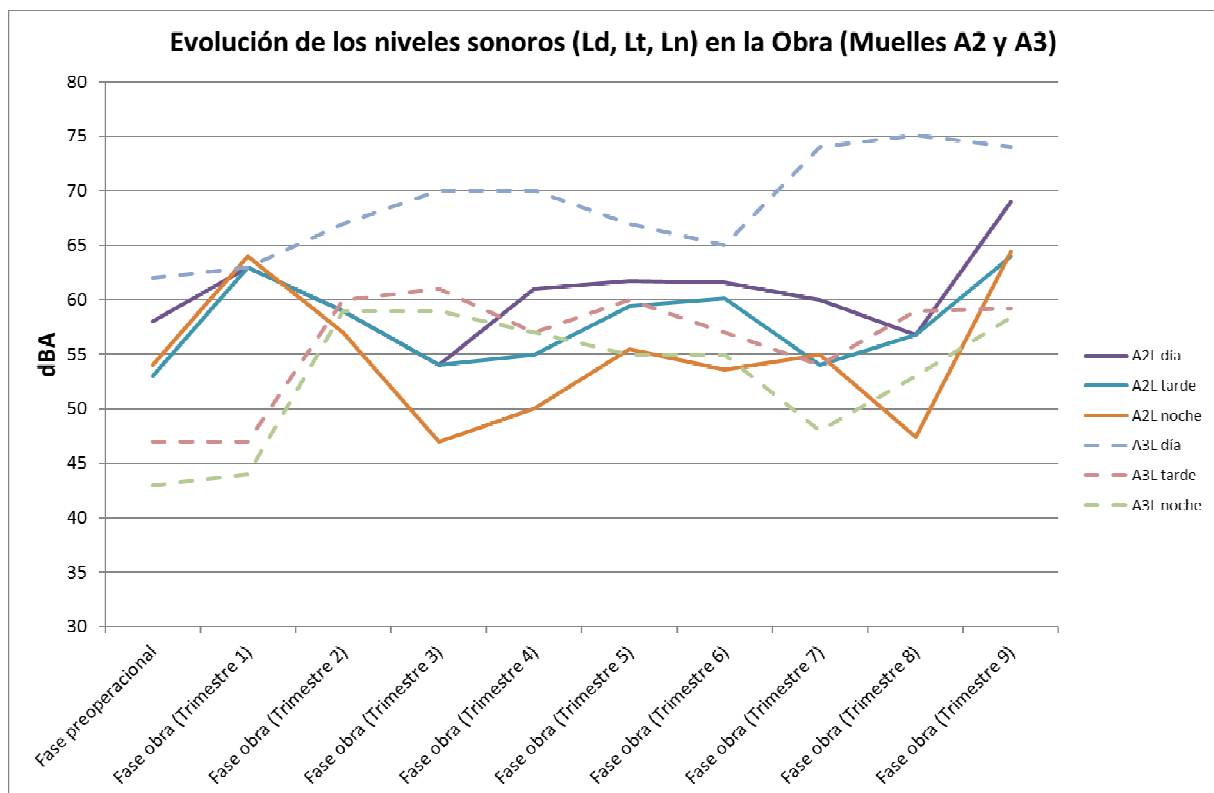
Figura 5. Evolución de los niveles de ruido en el desarrollo de la obra (Muelles)
